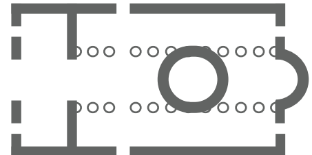
ΤΡΙΚΛΙΤΗ ΒΑΣΙΛΙΚΗ ΜΕ ΤΡΟΥΛΟ ΚΑΙ ΝΑΡΘΗΚΑ
